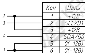
Схема кабеля 1 Розетка IDC-06F
