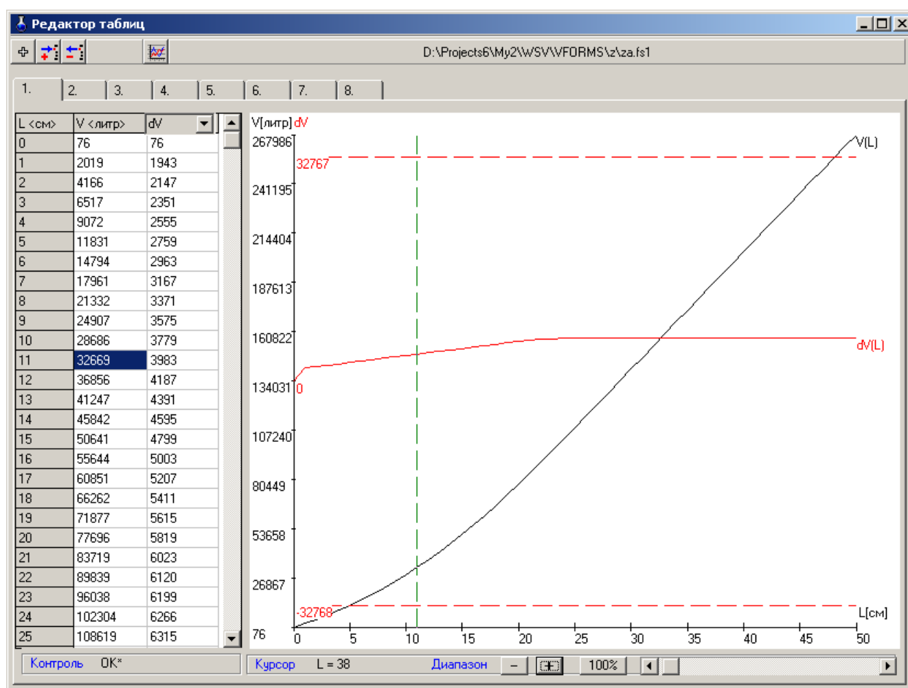
Рисунок 4.3 — Окно “Таблиц редактор” (коррекция “мёртвого остатка”)
